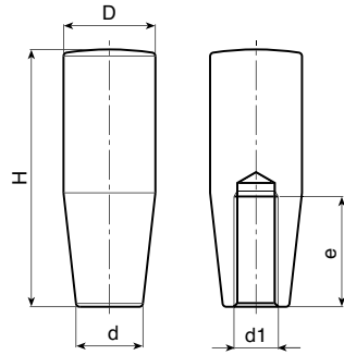
Agujero ciego con rosca directa. PA: Poliamida negra reforzada.
