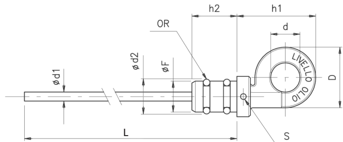
Versión 480084 - 2 juntas tóricas.
