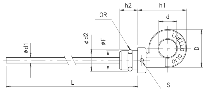
Versión 480082 - 1 junta tórica.
