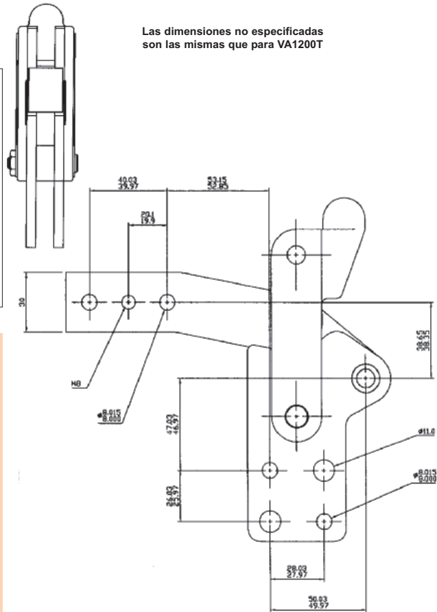
para mecanismo de bloqueo en "posición apertura" añade el sufijo (LC) al número de modelo
