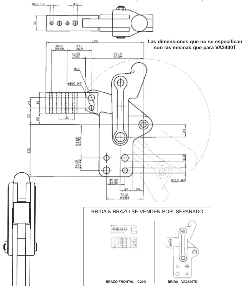
para mecanismo de bloqueo en "posición apertura" añade el sufijo (LC) al número de modelo
