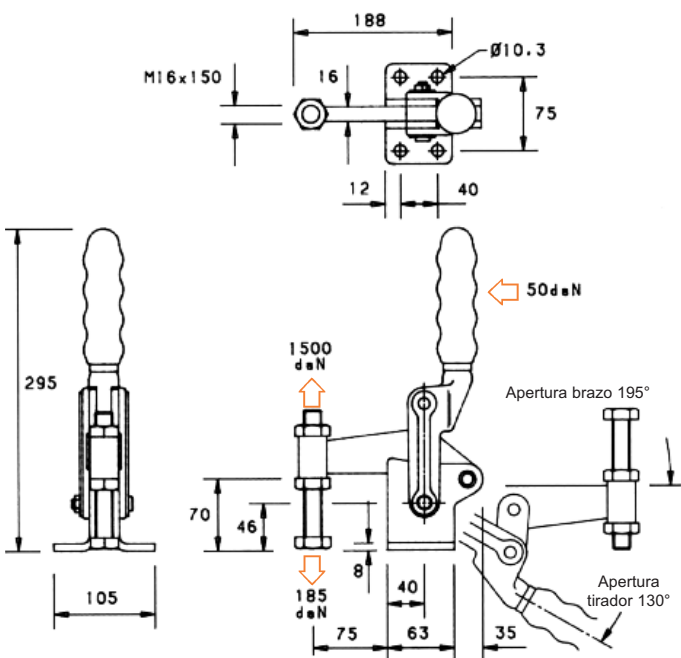
para mecanismo de bloqueo en "posición apertura" añade el sufijo (LC) al número de modelo
