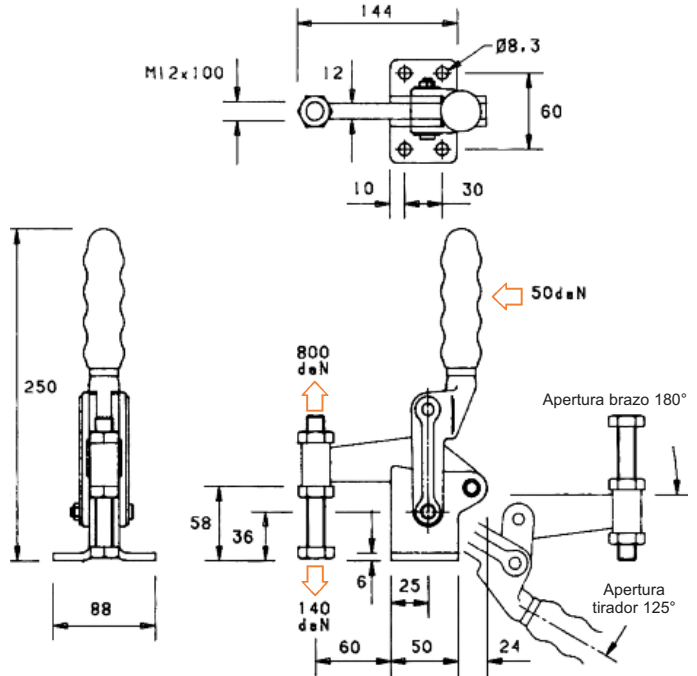
para mecanismo de bloqueo en "posición apertura" añada el sufijo (LC) al número de modelo
