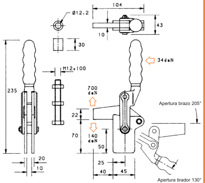
para mecanismo de bloqueo en "posición apertura" añade el sufijo (LC) al número de modelo
