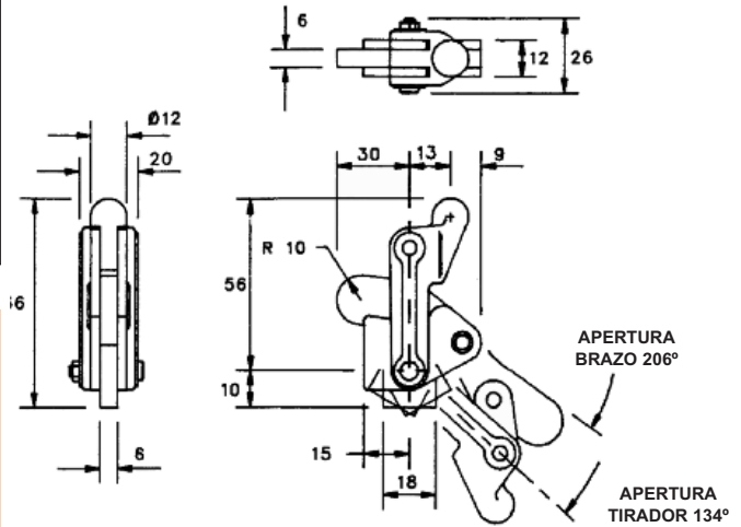
para mecanismo de bloqueo en "posición apertura" añade el sufijo (LC) al número de modelo
