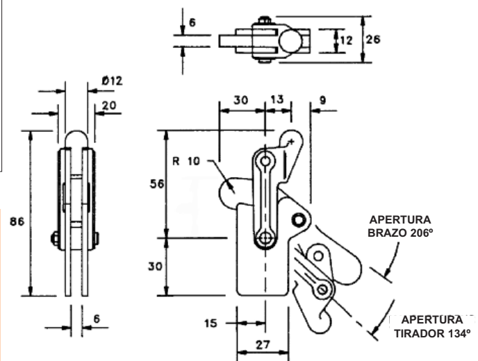
para mecanismo de bloqueo en "posición apertura" añade el sufijo (LC) al número de modelo
