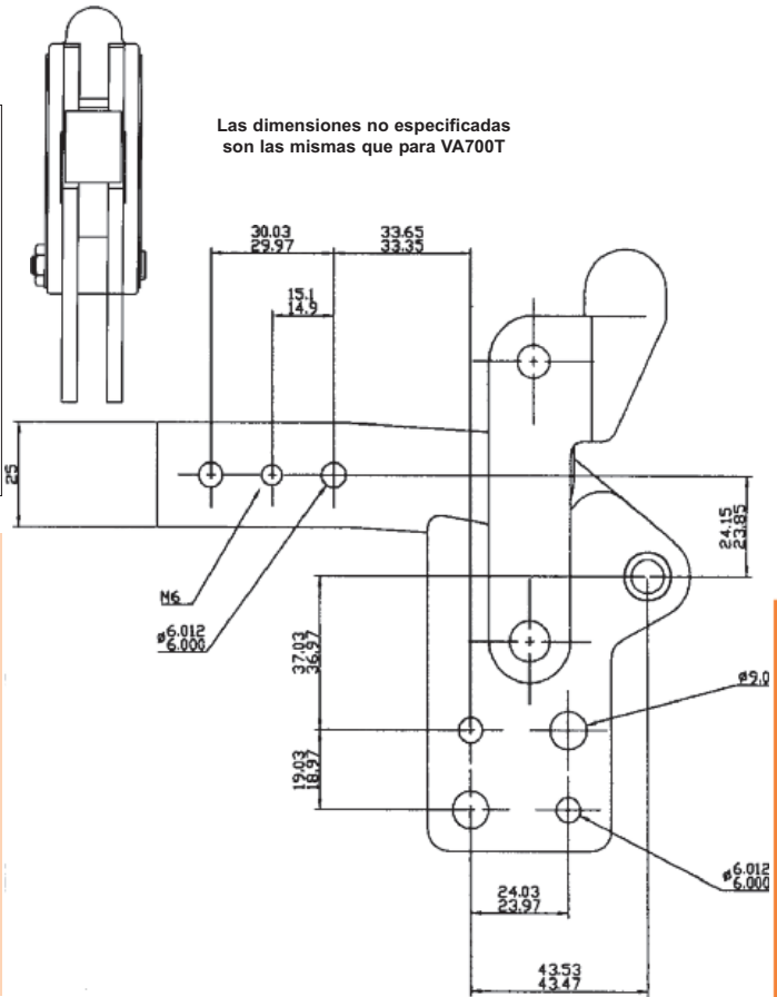
para mecanismo de bloqueo en "posición apertura" añade el sufijo (LC) al número de modelo
