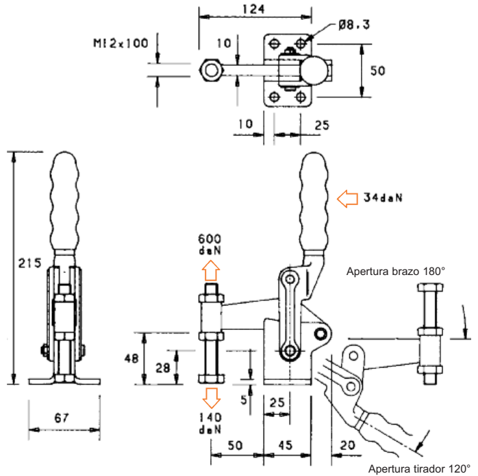
para mecanismo de bloqueo en "posición apertura" añade el sufijo (LC) al número de modelo
