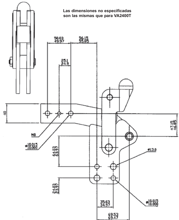
para mecanismo de bloqueo en "posición apertura" añade el sufijo (LC) al número de modelo
